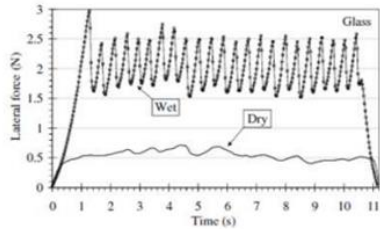
Zmiana siły tarcia szkła i PP po skórze (na sucho i na mokro) R=20\text{ mm} , F_n=2\text{ N} , v_s=8\text{ mm/s}
